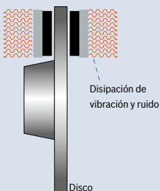
Pastilla convencional
